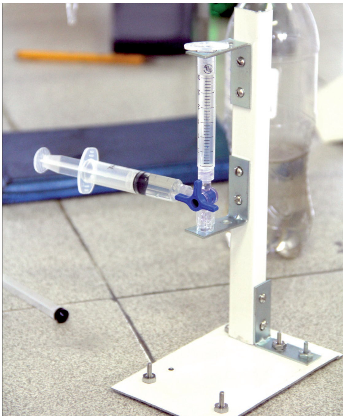
Microbureta elaborada con jeringas y otros implementos
